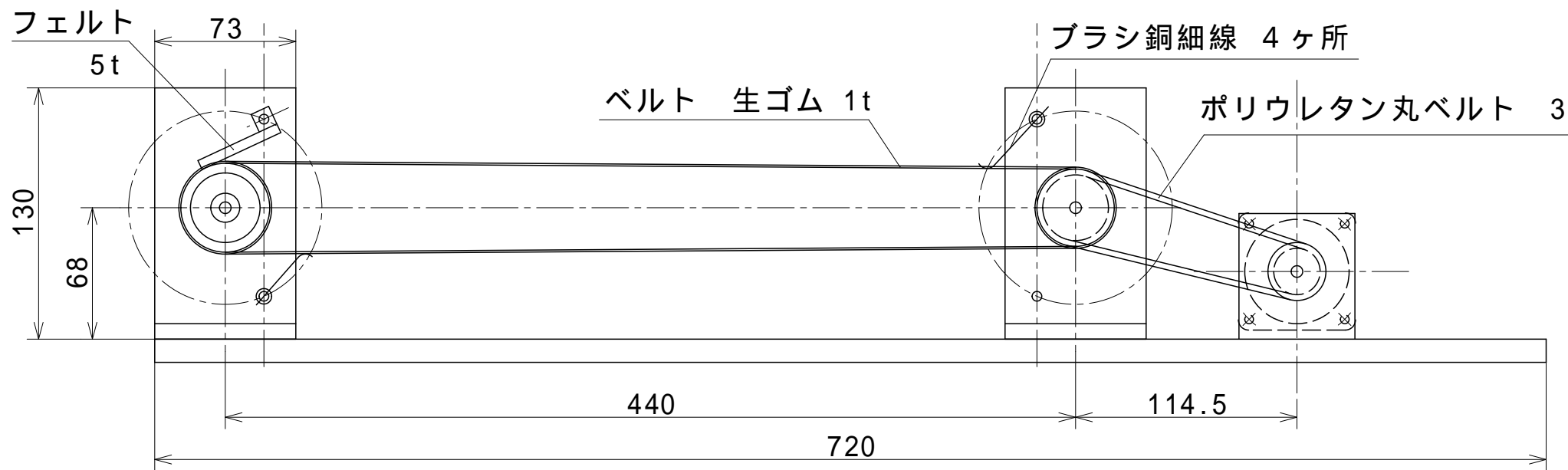
ベルト式静電発電機 S = 1 / 3
