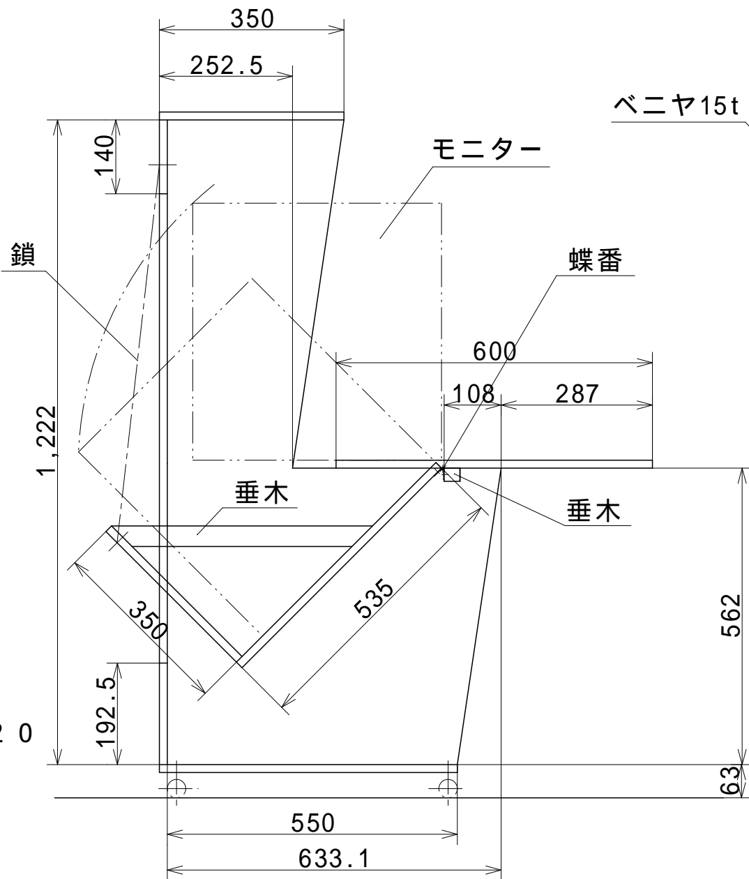
パソコンデスク S = 1 / 1 0
