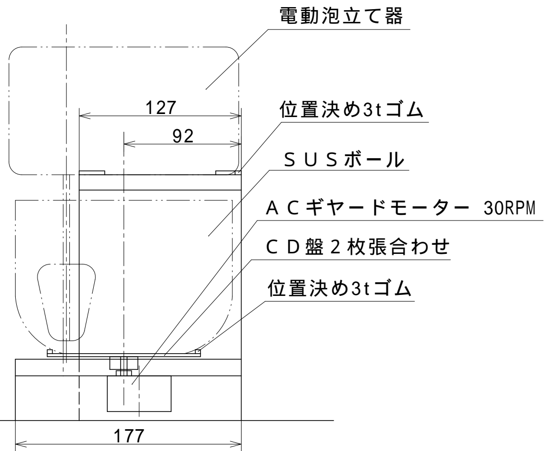
自動泡立て器 S = 1 / 3
